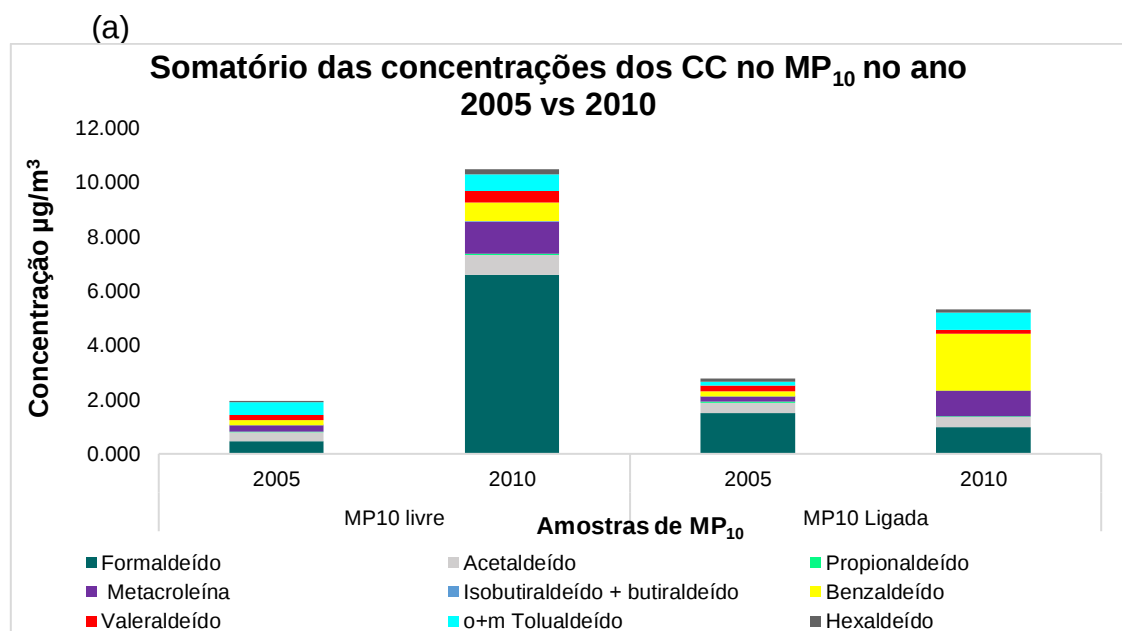
Figura 32. Somatório das concentrações dos CC no MP 10 no ano 2005 vs 2010.
