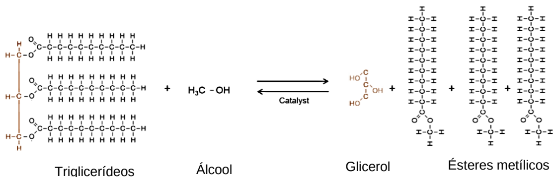
Figura 9. Reação de triglicerídeos no processo de transesterificação para produzir ésteres metílicos como combustível biodiesel (PEREIRA et al., 2002)
