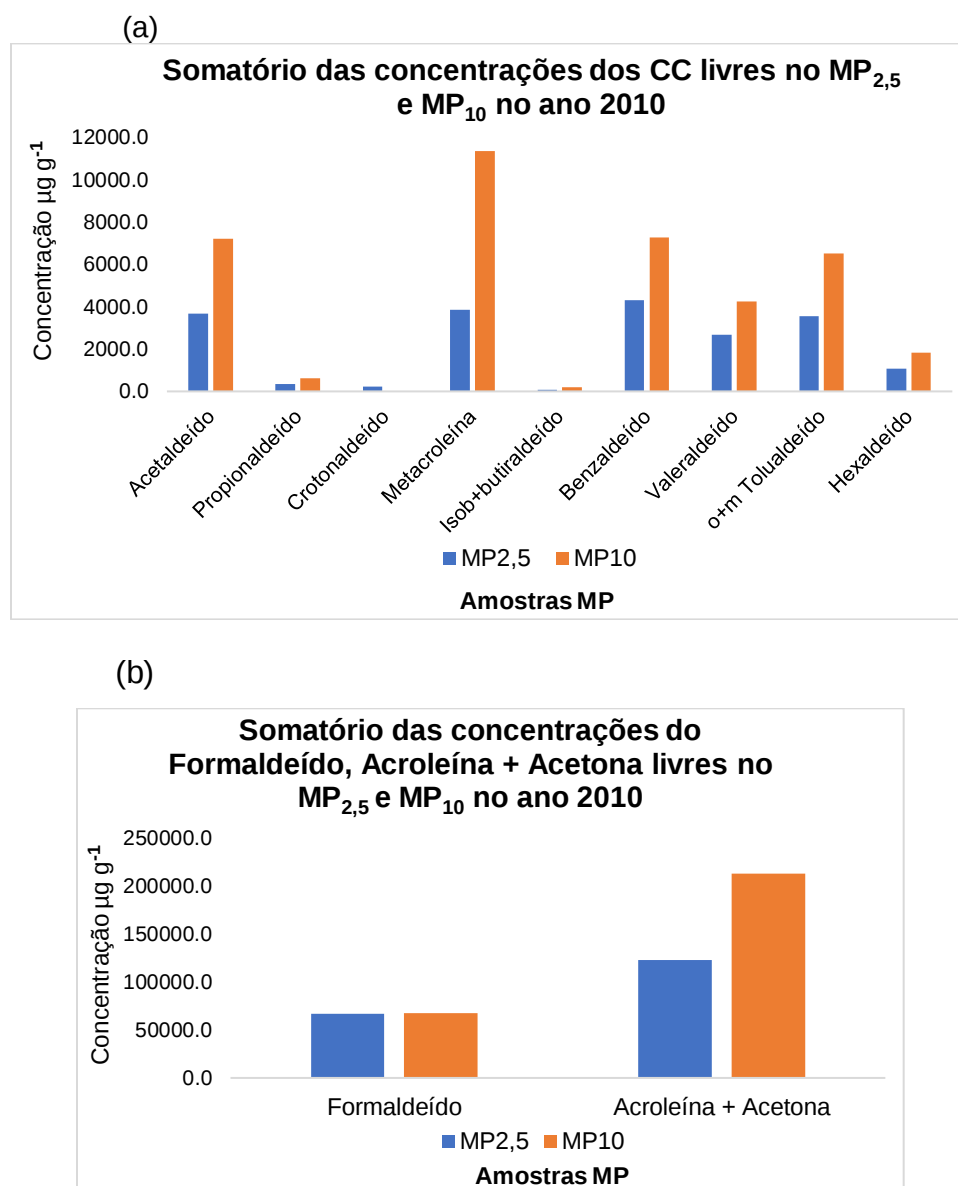
Figura 40. Somatório das concentrações em \mu\text{g g}^{-1} dos CC livres no \text{MP}_{2,5} e \text{MP}_{10} no ano 2010
